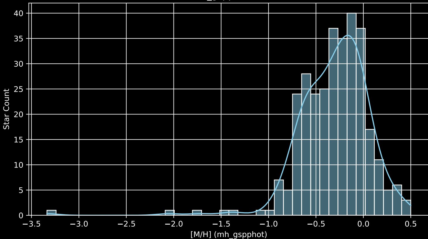
GALAH DR4 Field: [7004] [M/H] (mh_gspphot) (n= 311)
