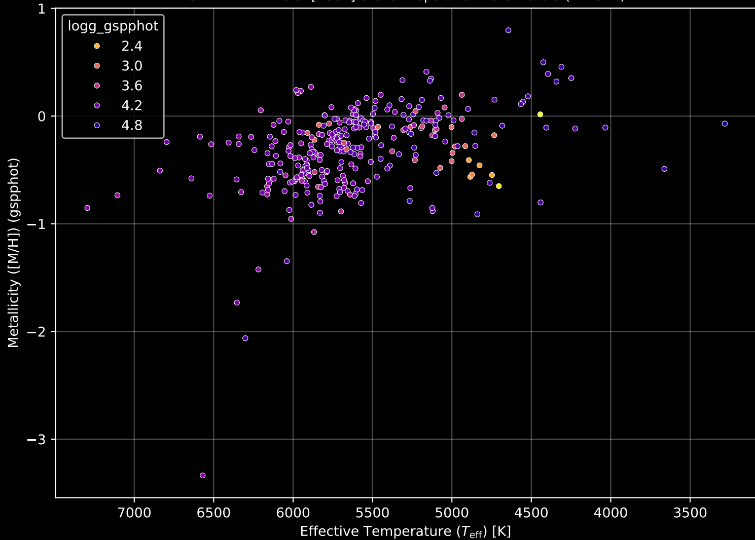
GALAH DR4 Field: [7004] Stellar Population Parameters (n= 312)
