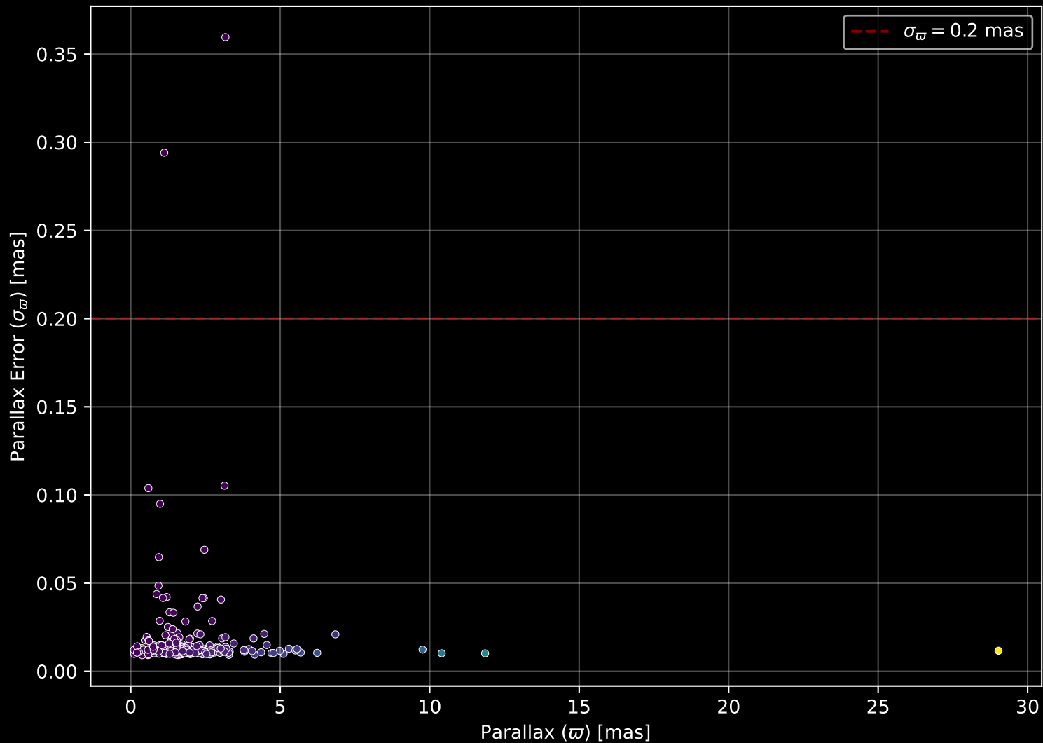
GALAH DR4 Field: [7004] Parallax Quality (n= 312)
