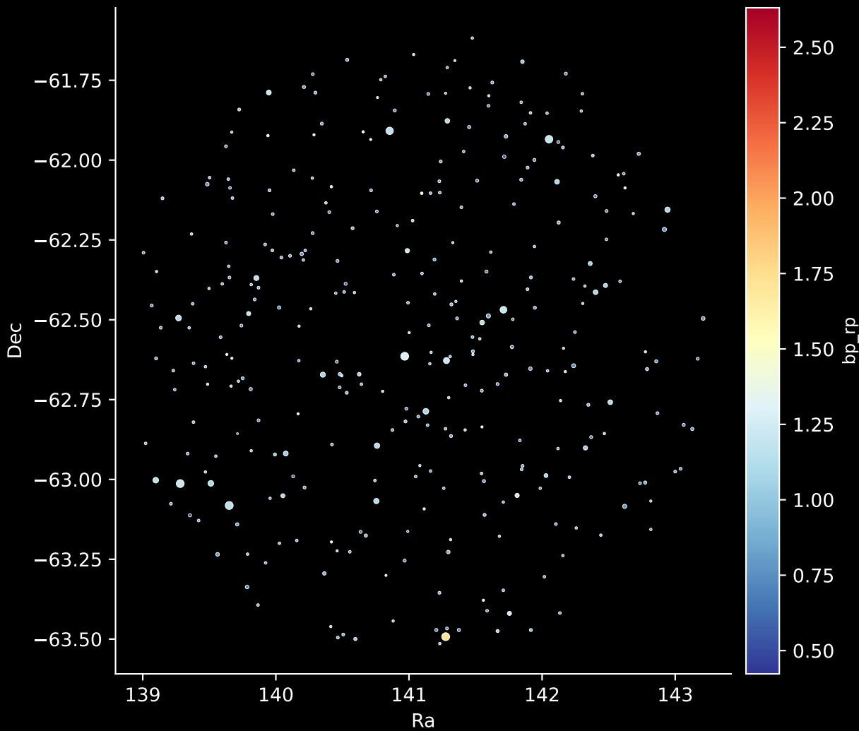
GALAH DR4 Field: [7004] Stars: 312
